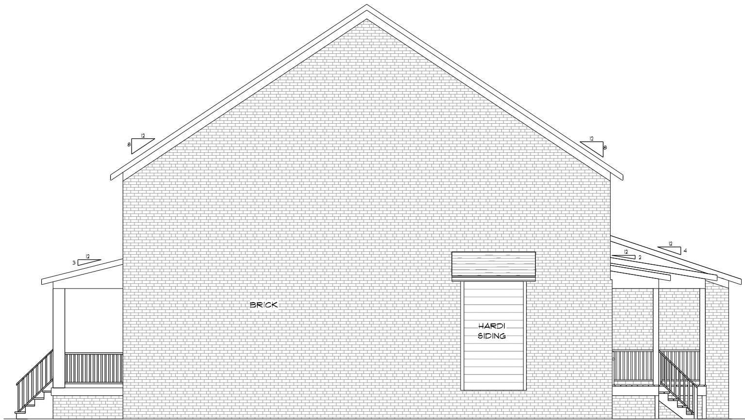
RIGHT ELEVATION
